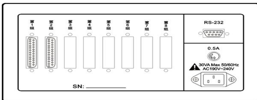
图4 后面板
