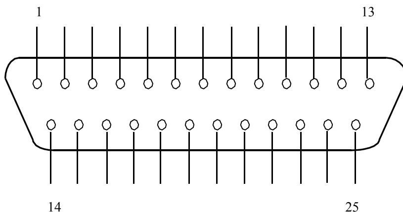
温度测试盒接口引脚示意图
