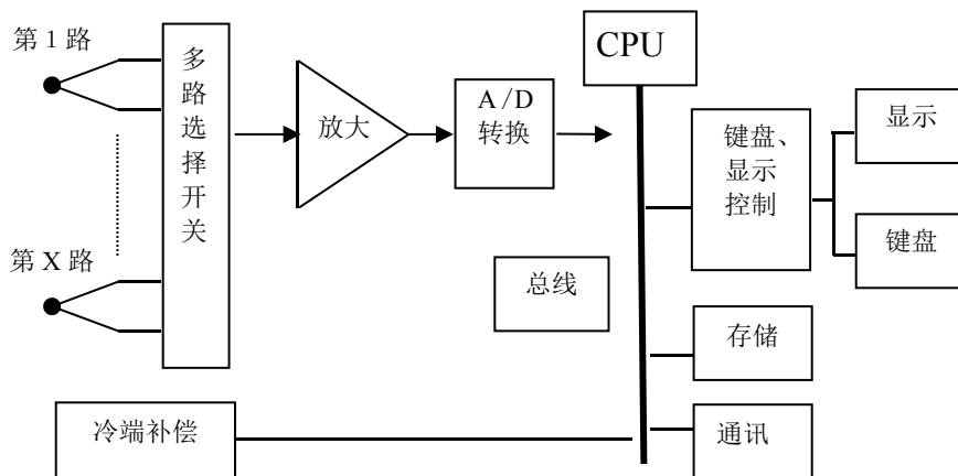
原理框图
